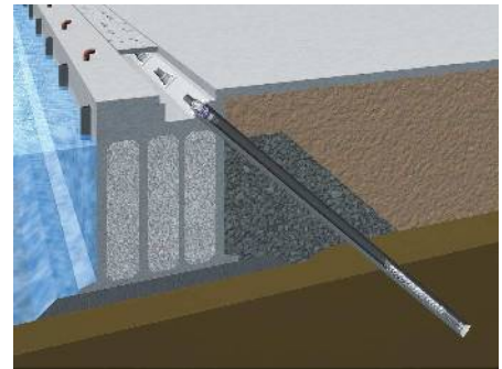
<岸壁・護岸補強アンカー工法>
